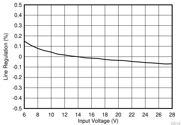
图 7-3. 线性调整率
