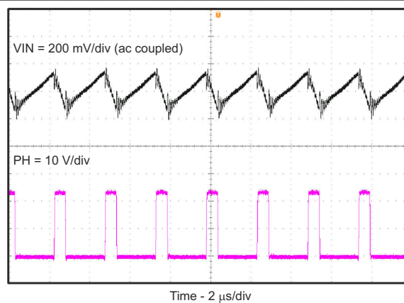
图 7-5. 输入电压纹波
