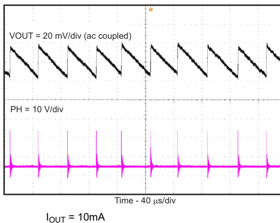
图 7-7. 输出电压纹波
